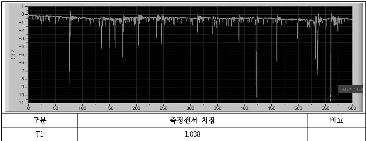
【그림 6.2】 교량의 처짐 측정 DATA
