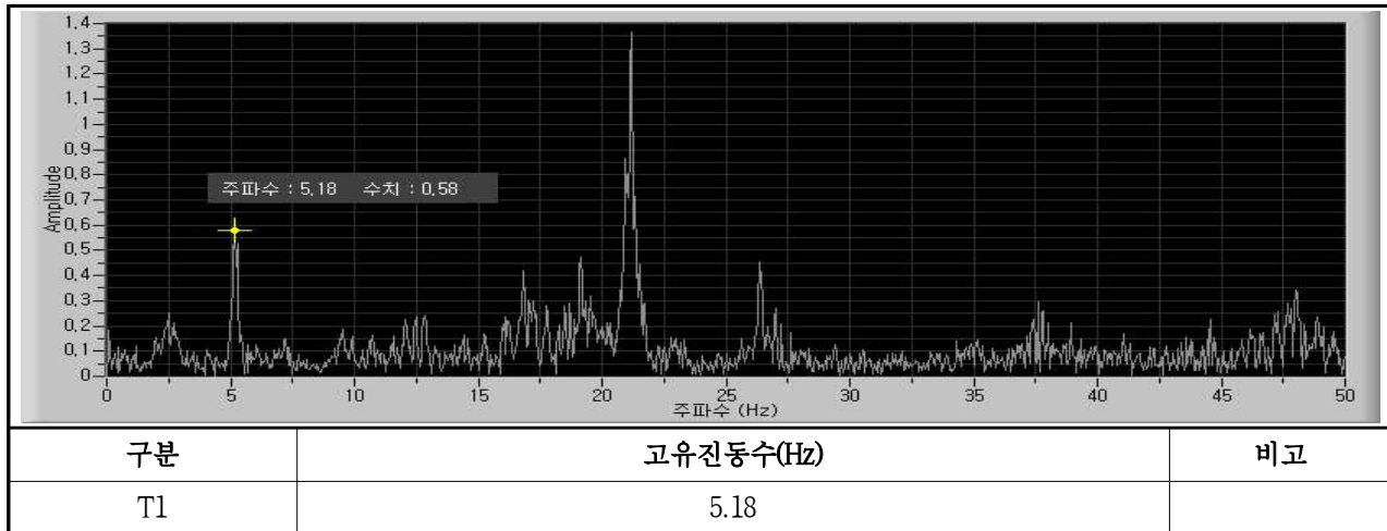
【그림 6.5】 교량의 고유진동수 측정 DATA
