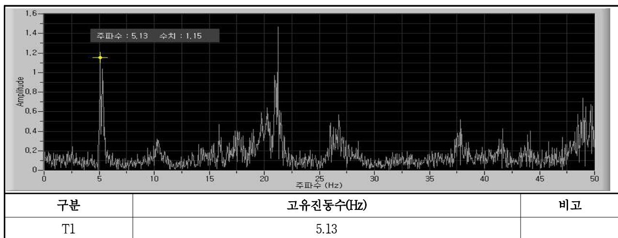
【그림 6.3】 교량의 고유진동수 측정 DATA
